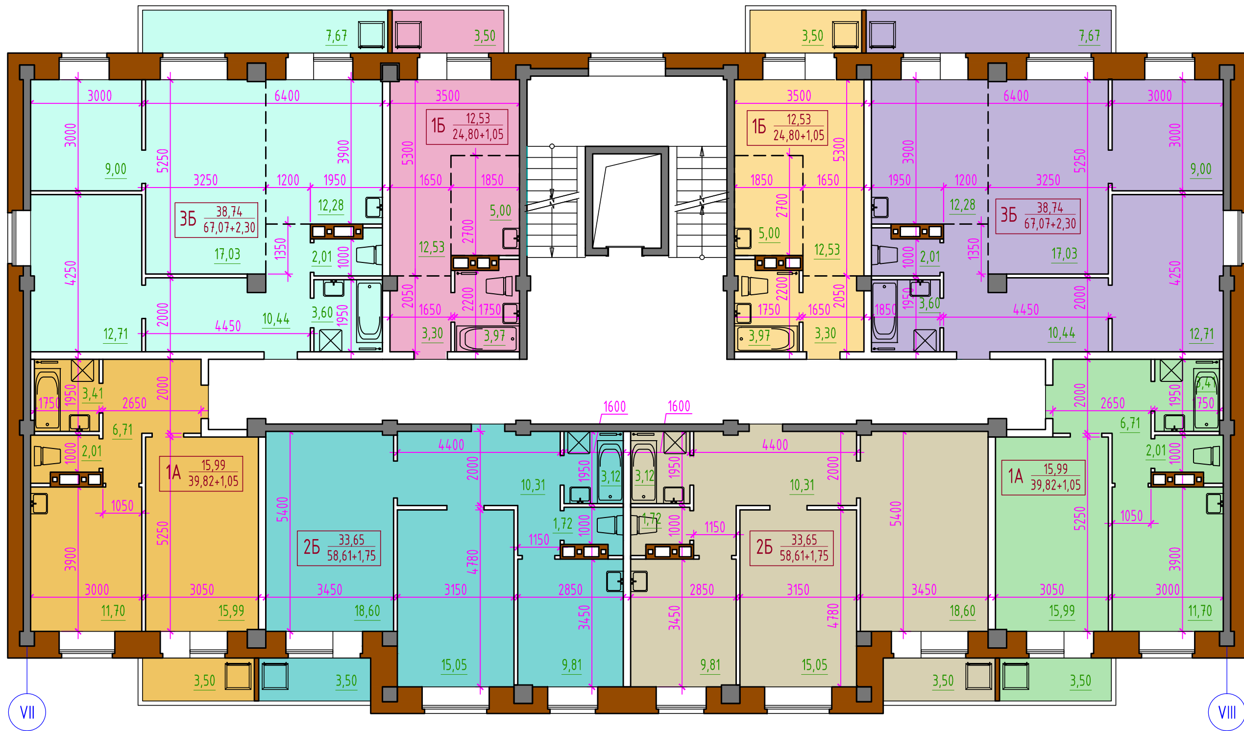
План 2-9 этажа блок-секции в осях VII-VIII
